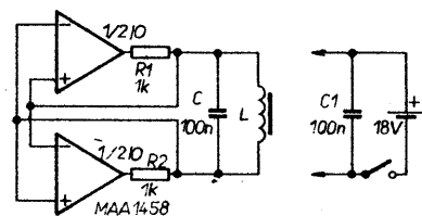
Obr. 3. Úprava zapojení z obr. 1
